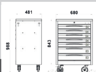
DIMENSIONI CASSETTO FG 102
