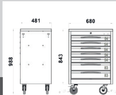
DIMENSIONI CASSETTO FG 104
