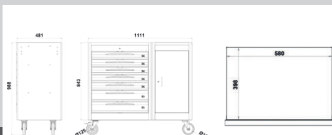
DIMENSIONI CASSETTO FG 105
